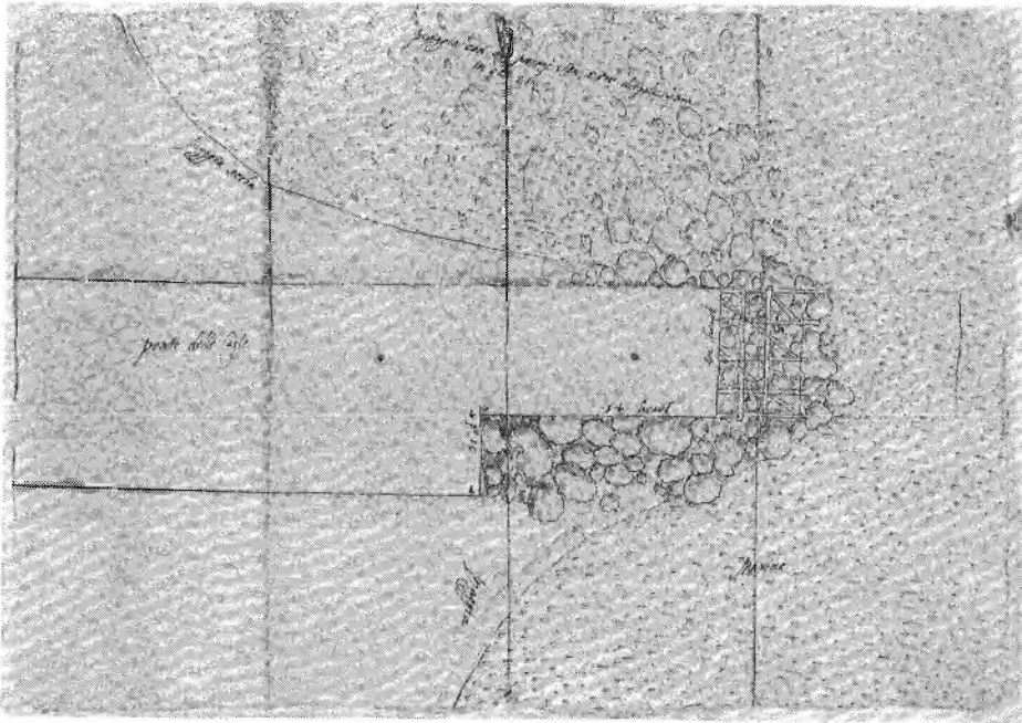
Fig. 9 - Disegno del «gagiolo» al molo delle Casse . 1603. Disegno a inchiostro su carta, mm 297 x 424, Genova, Archivio di Stato, Senarega, 1660.
