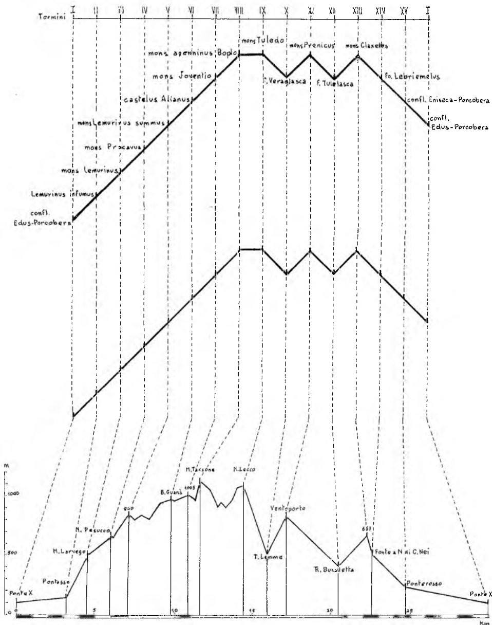
Fig. 3 - Profili altimetrici reale e schematico dei nuovi confini dell'agro pubblico comparati col profilo altimetrico schematico ricavato dal testo della Sentenza.
